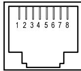
Schéma du connecteur 10BT (face arrière du modèle 55)
