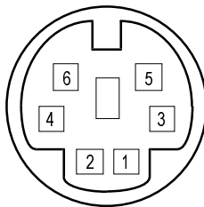
Connecteur clavier (face arrière du modèle 55)
